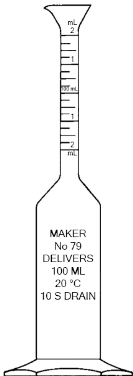
Fig. 1. 100 mL glass flask.
